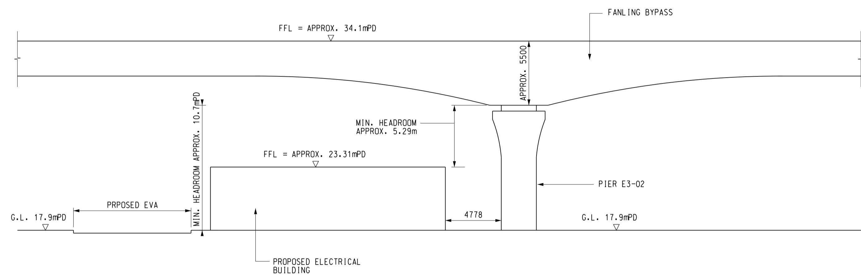
SECTION 03 SCALE 1 : 200 AIS-002
