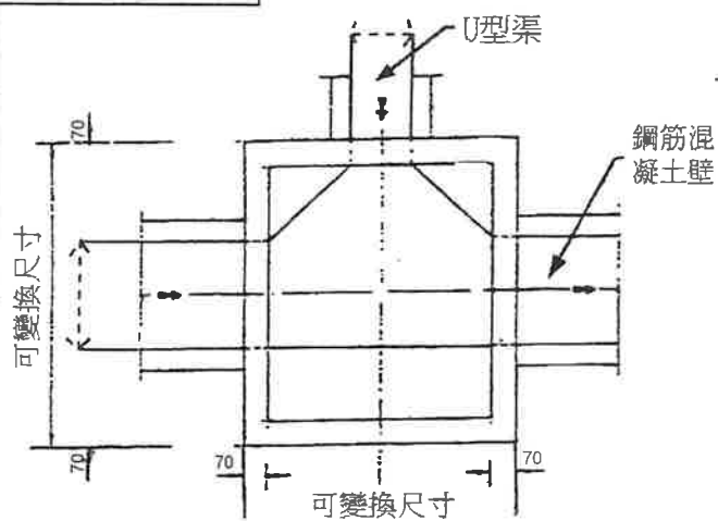
沙井俯視圖
