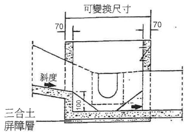
沙井切面圖
