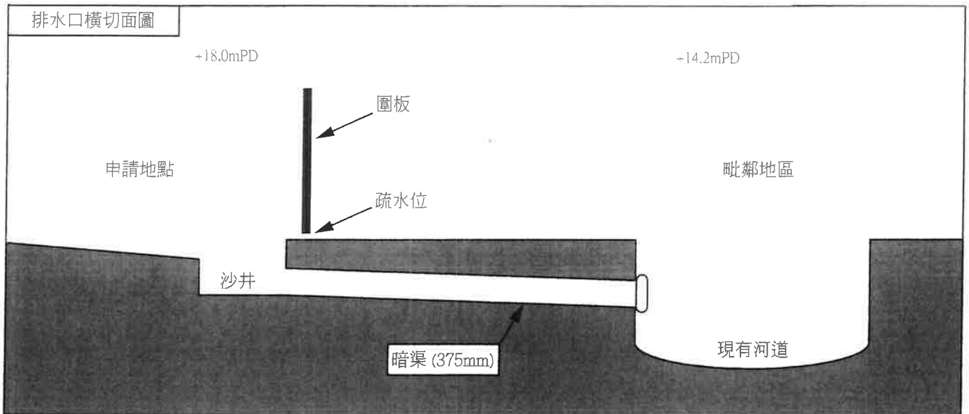
U型明渠橫切面圖
