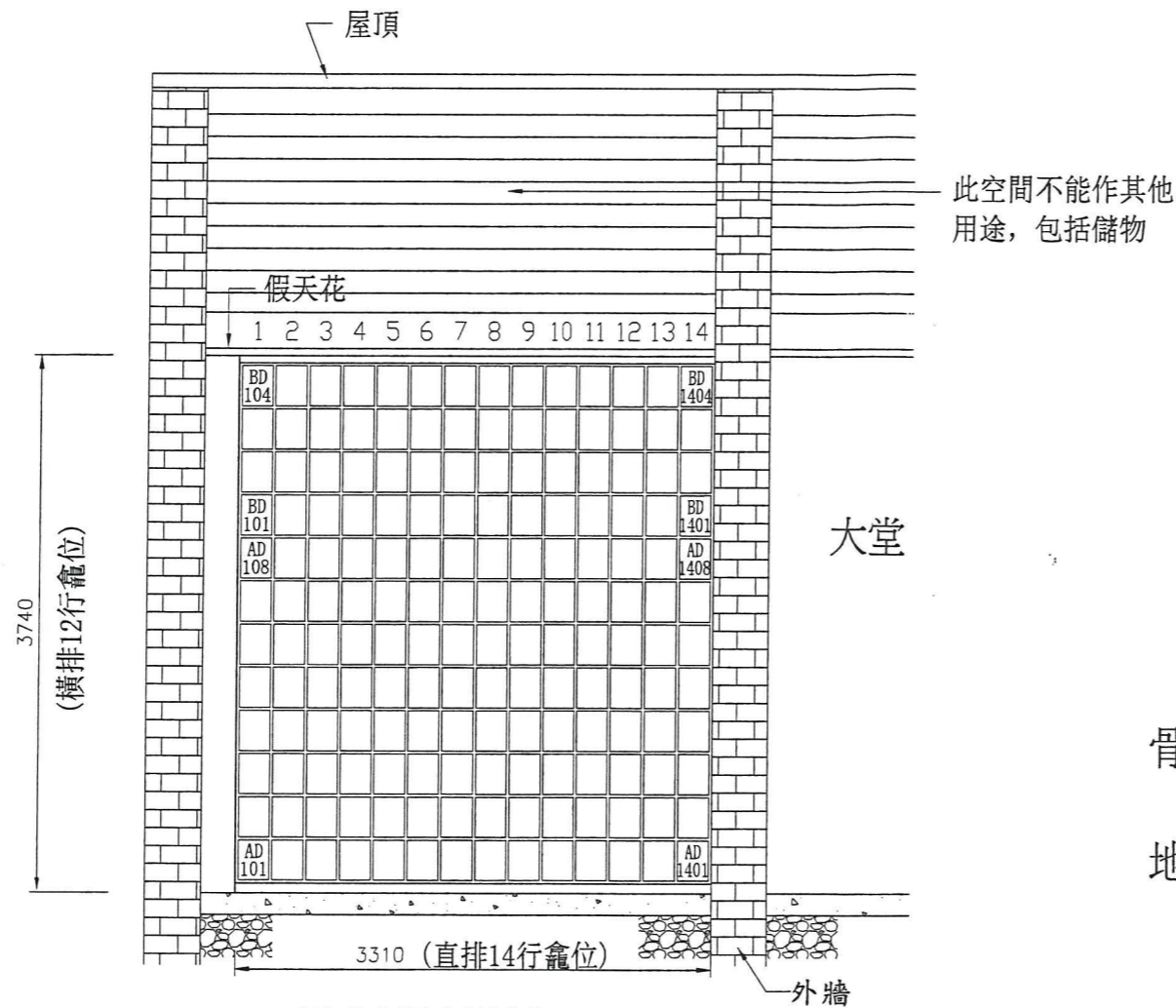
龕牆4 建議骨灰安置所大樓樓面立面圖 (圖則編號003D)
