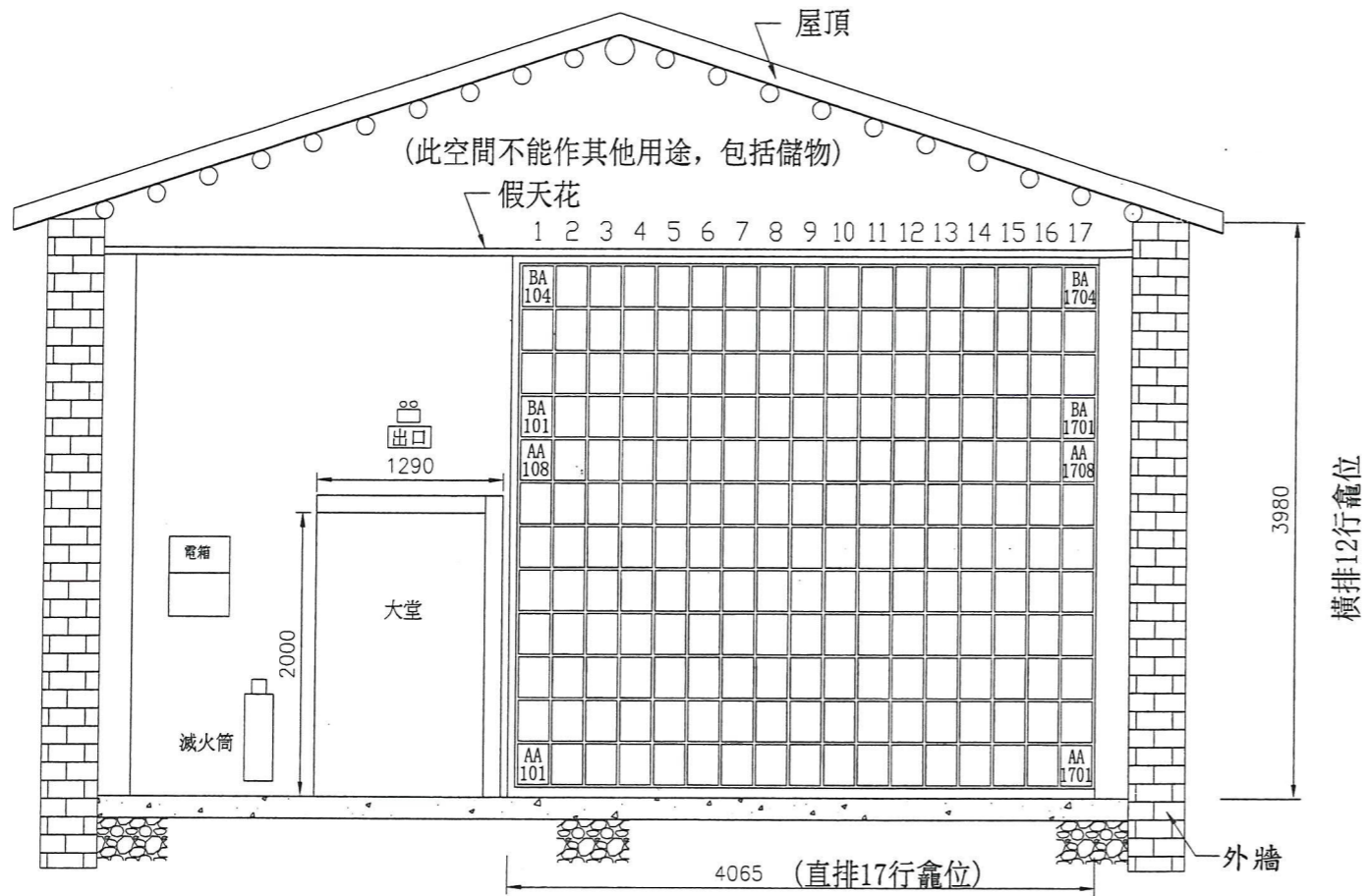
龕牆1 建議骨灰安置所大樓樓面立面圖 (圖則編號003A)
