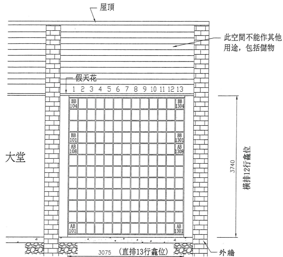
龕牆2 建議骨灰安置所大樓樓面立面圖 (圖則編號003B)
