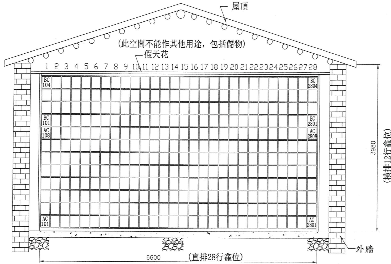
龕牆3 建議骨灰安置所大樓樓面立面圖 (圖則編號003C)
